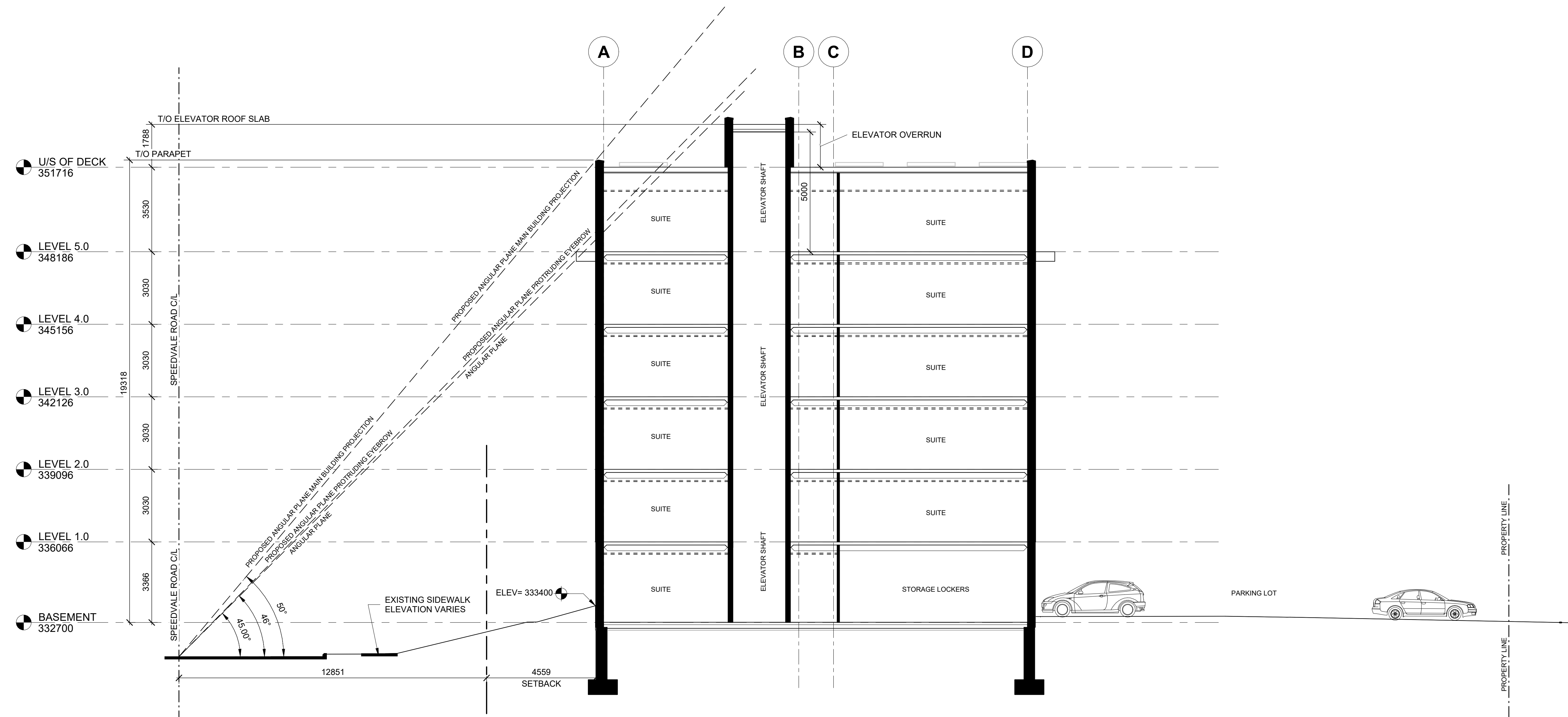
1 CROSS SECTION SCALE: 1 : 100
